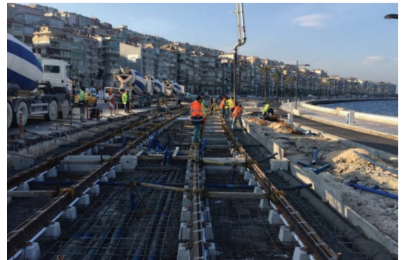
Konak Tramvayı Mustafa Kemal Sahil Bulvarı Hat İmalatı
